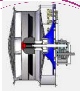
Fan unit
