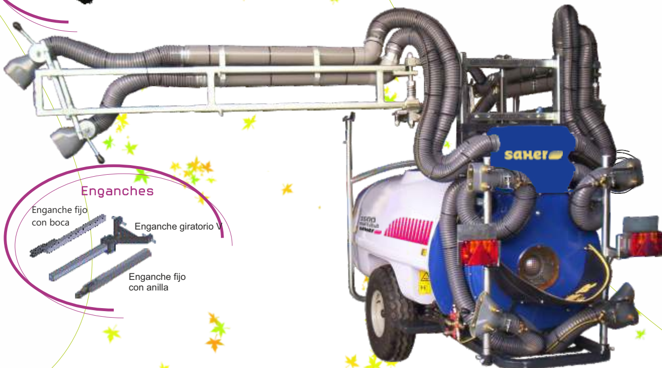
Movimiento brazos hidráulicos: subir/bajar; abrir/cerrar individual.
